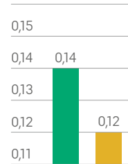
Traction perpendiculaire à l'eau bouillante en N/mm²
